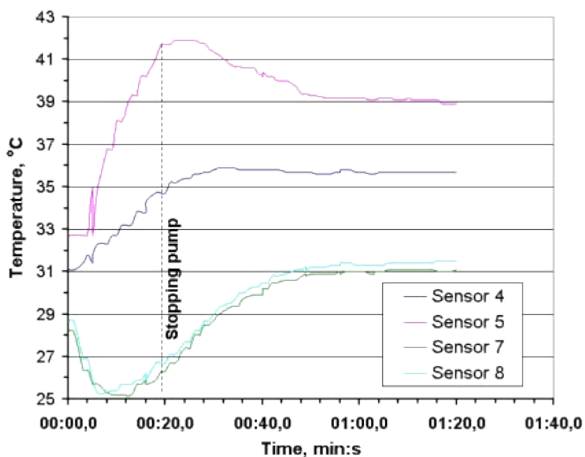
Рис. 3. Эффект перетекания тепла от холодного тела к горячему при прохождении водяной смеси через специальный вихревой кавитатор, датчик 8 - температура стенки трубы сразу после кавитатора, датчик 5 - температура воды в этом месте, датчик 7 - температура стенки трубы на отдалении от кавитатора, датчик 4 - температура воды в этом месте
